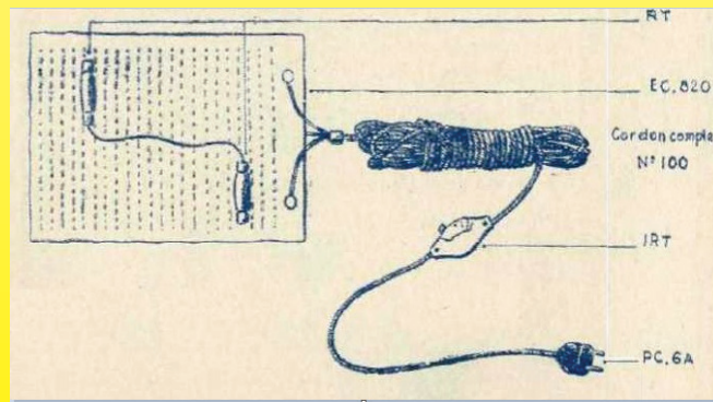
1947 Термоплазм Calor, вид на нагревательную часть с двумя термостатами в защищенной оболочке (RT) и трехпозиционным переключателем (IRT). (Cat Ultiheat)
