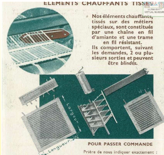
1939 Асбестовые тканые элементы (Каталог Noiro 1939, Музей Ultimheat)
