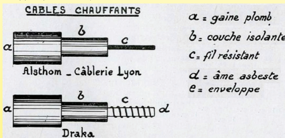
Греющие кабели Alsthom, Câblerie de Lyon, Draka (1938 защищенные элементы, Gautheret, Музей Ultimheat)
