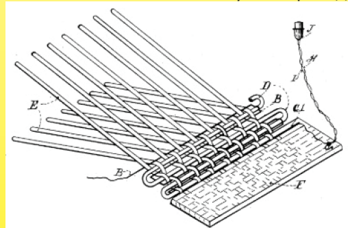
4 июня 1895 года, США. Патент №. 540398, Джон Эмори Мик из Денвера, для компании “Джонс Мэнүфэчуринг Сай” из Нью-Йорка, описал нагревательную ткань, нити основы которой (E) изготовлены из асбеста, а уточные пряжи (B) - из проводящего металла, со второй асбестовой прослойкой ткани (D). Два конца нагревательного элемента (F) не включают нагревательный провод.
